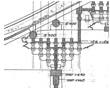
산청 율곡사 대웅전 공포 (출처 : 국가유산청)
