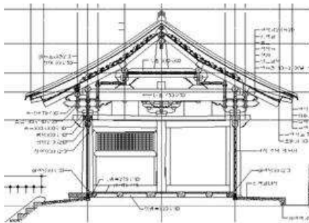
안동 광흥사 응진전 종단면도
