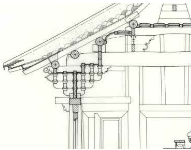
청도 대비사 대웅전 공포 (출처 : 국가유산청)
