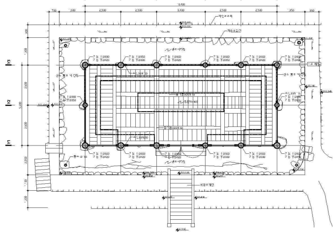
안동 광흥사 응진전 평면도 (출처 : 지정신청보고서)
