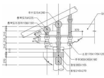
안동 광흥사 응진전 공포 (출처 : 지정신청보고서)
